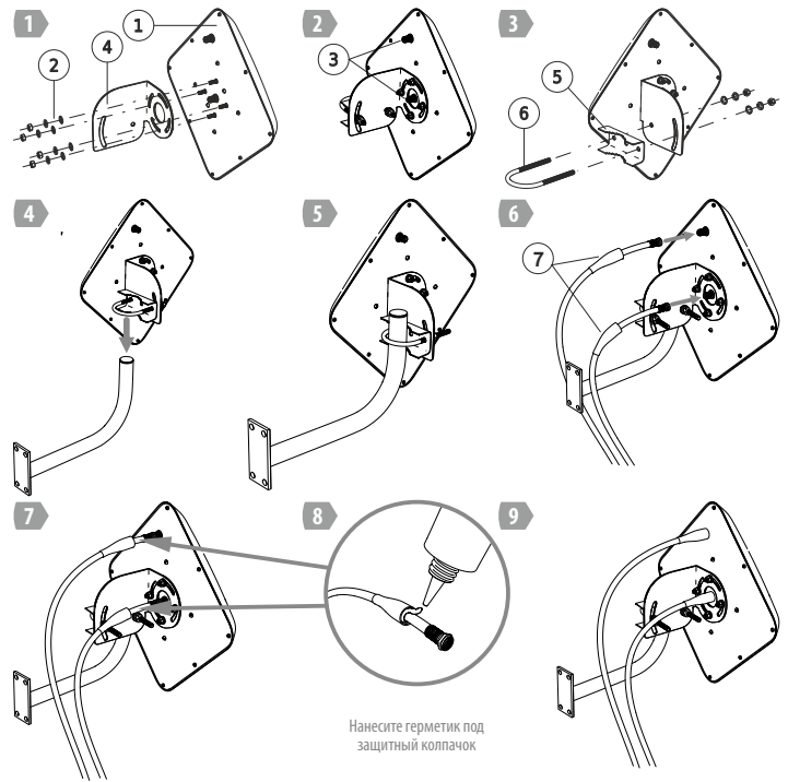
Рисунок 2. Узлы антенны и сборка BAS-2325 «Connect Street Direct 3G/4G»
