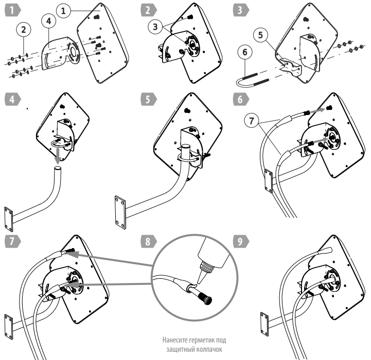
Рисунок 2. Узлы антенны и сборка BAS-2325 «Connect Street Direct 3G/4G»
