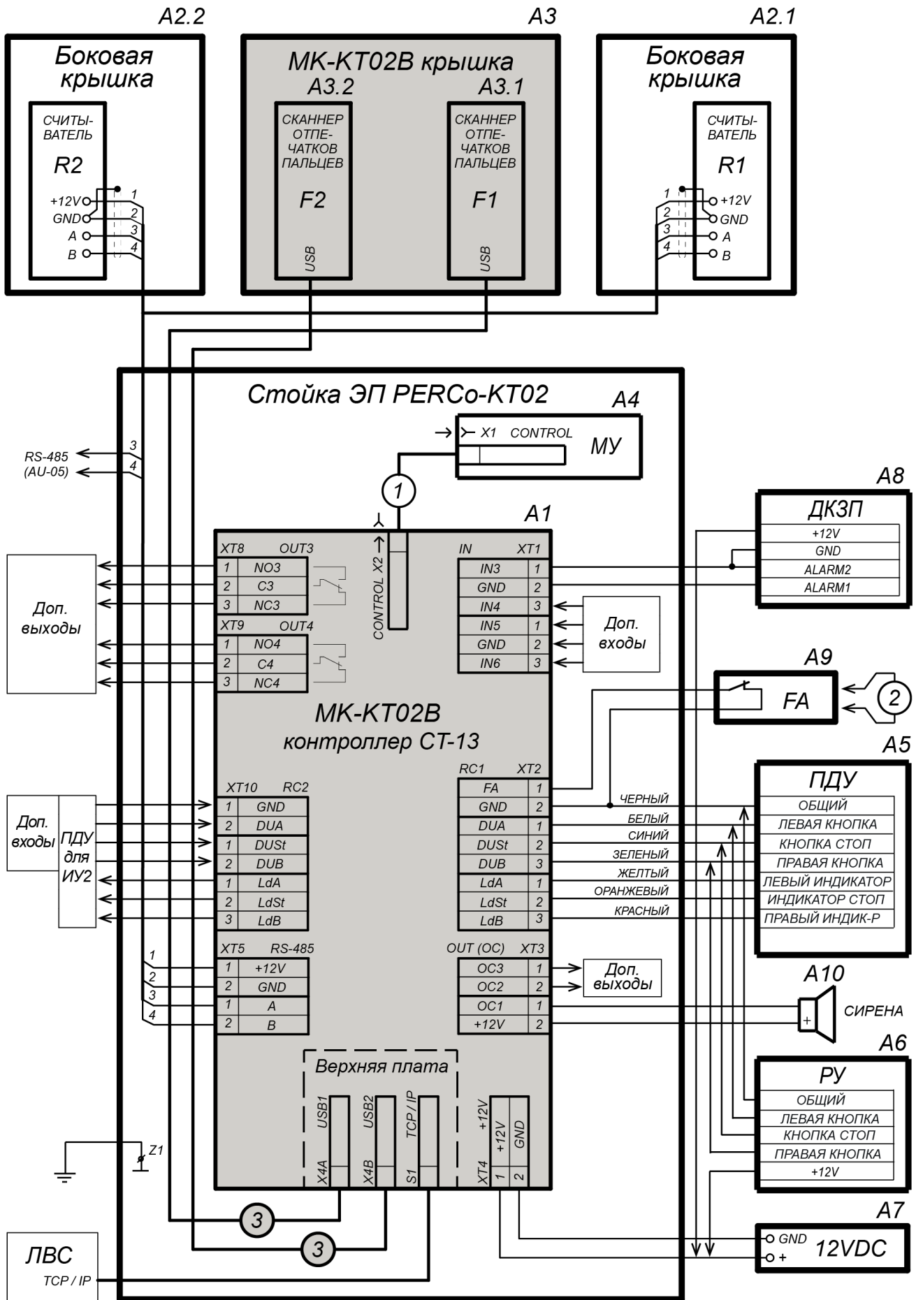
Рисунок 2. Схема подключения контроллера PERCo-CT13 к ЭП типа PERCo-KT02 (серым цветом выделены элементы монтажного комплекта PERCo-МК-КТ02В)
