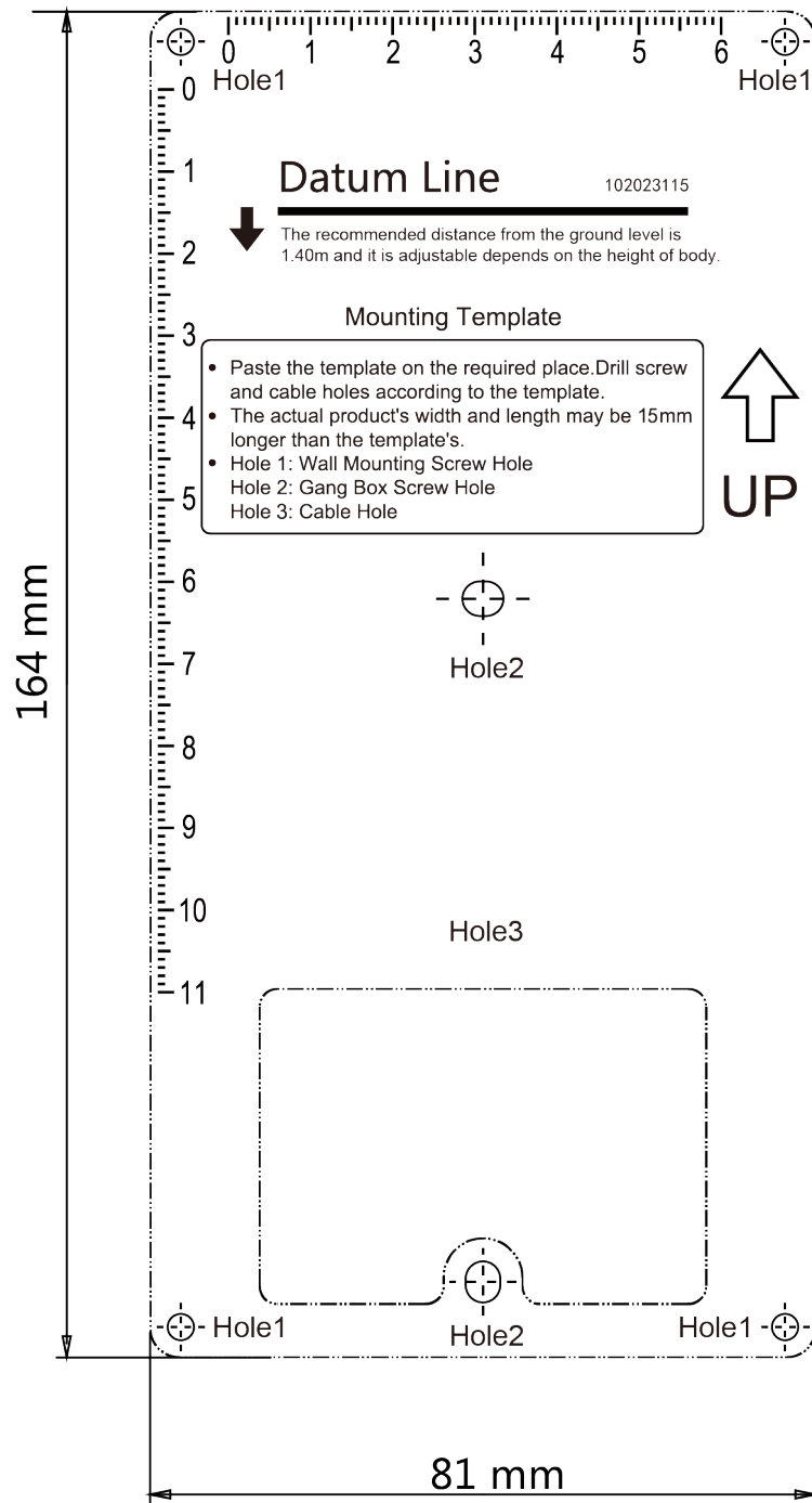
Рисунок 3-2. Монтажный шаблон
