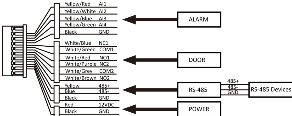
Рисунок 2-1. Описание разъемов
