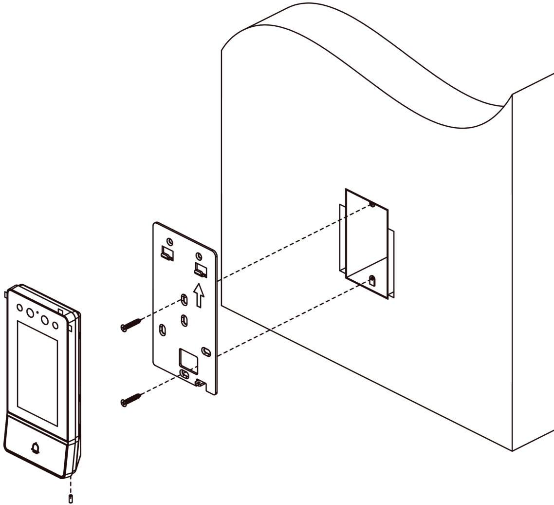
Рисунок 3-4. Врезная установка
