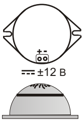
Рис.2 Схема подключения и диаграмма направленности оповещателя.
