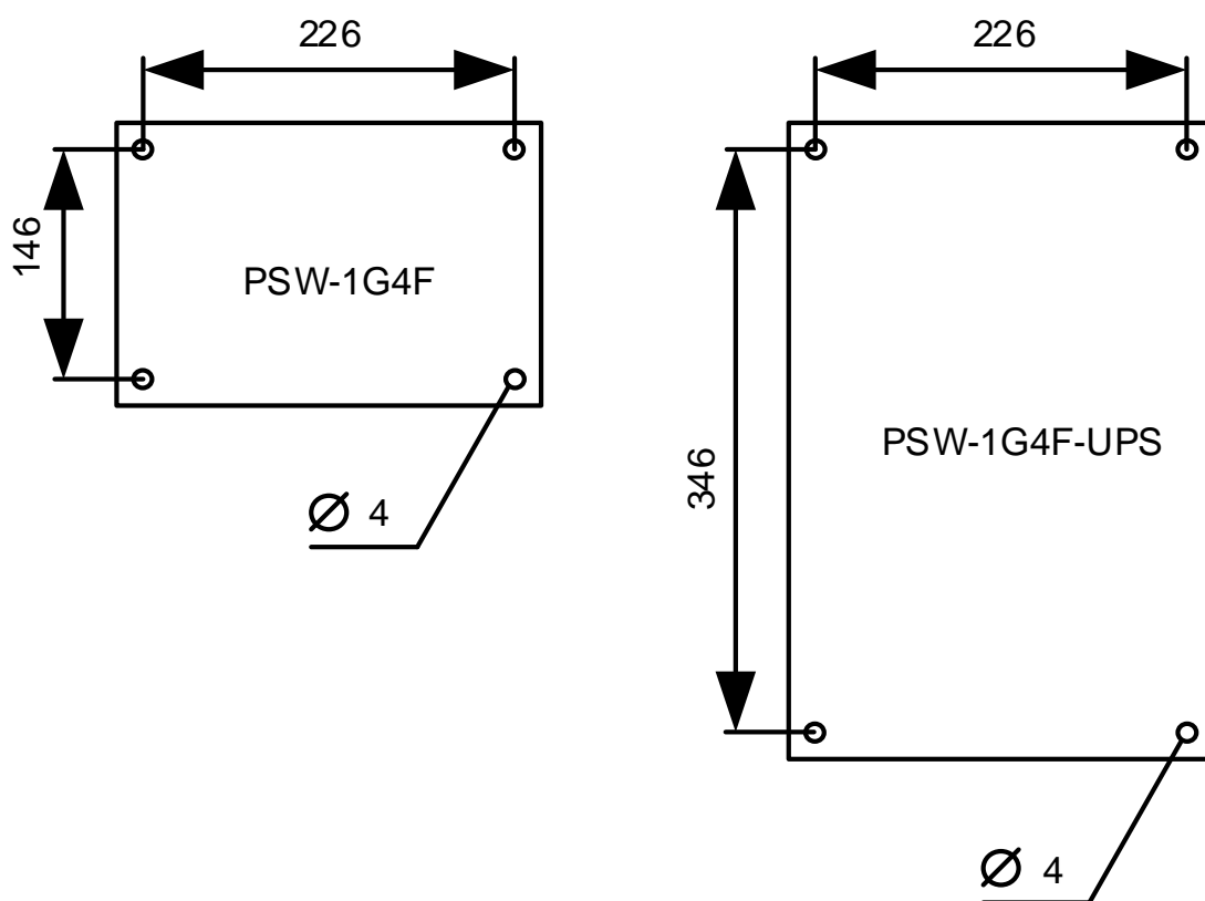
Рис. 6.1.1. Разметка крепления
