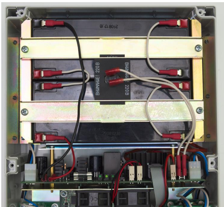
Рис. 2.9.5. Подключение АКБ.
