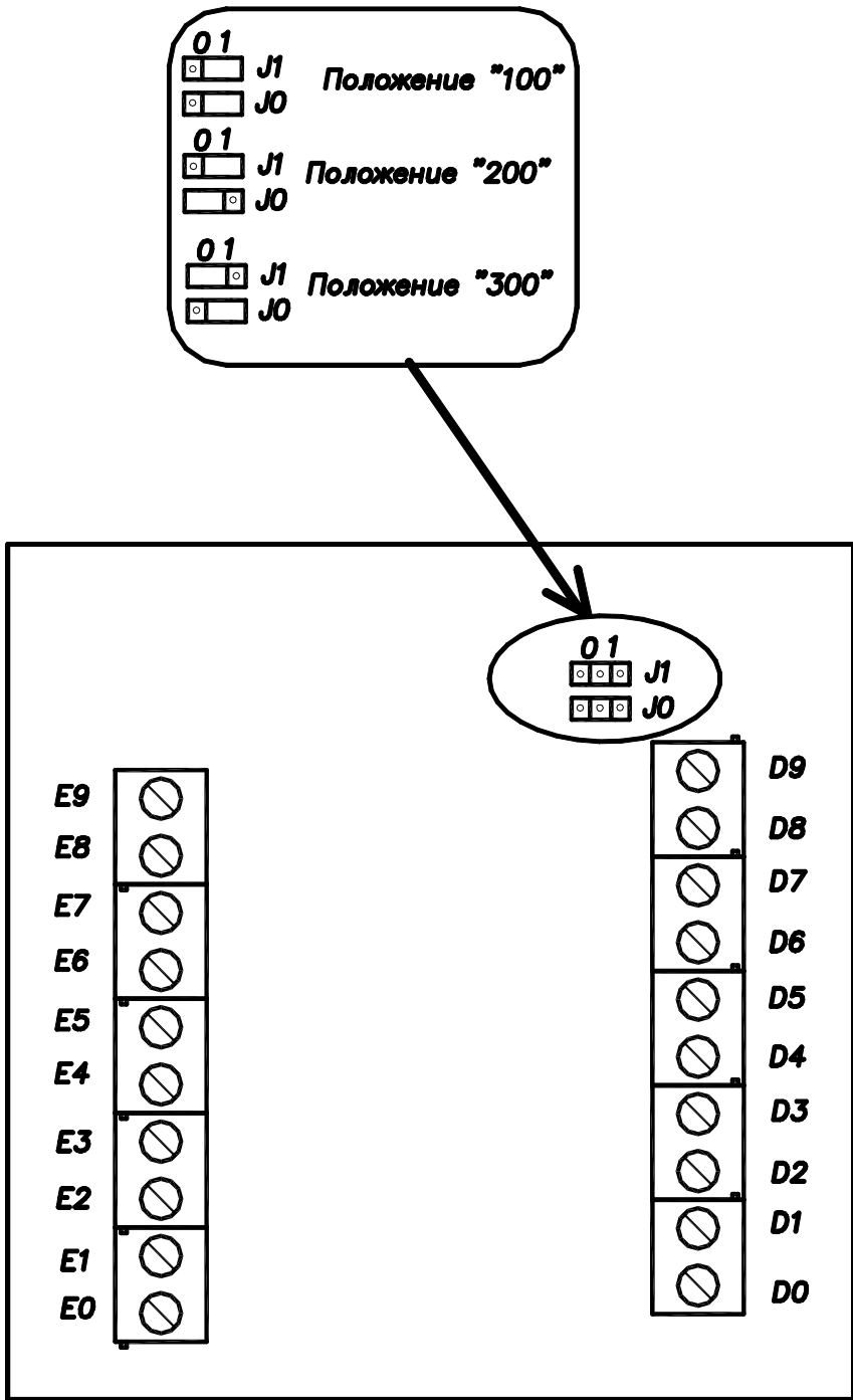
Рис4. Установка джамперов в коммутаторе KM100-7.3
