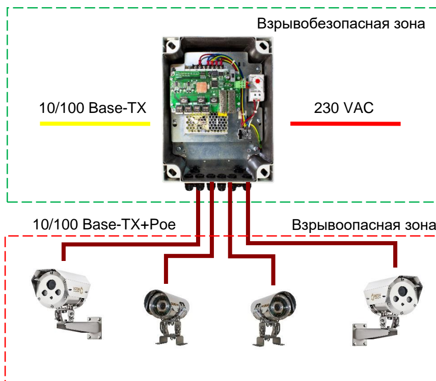
Рисунок 2. Типовая схема подключения коммутаторов по одному оптическому кабелю.
