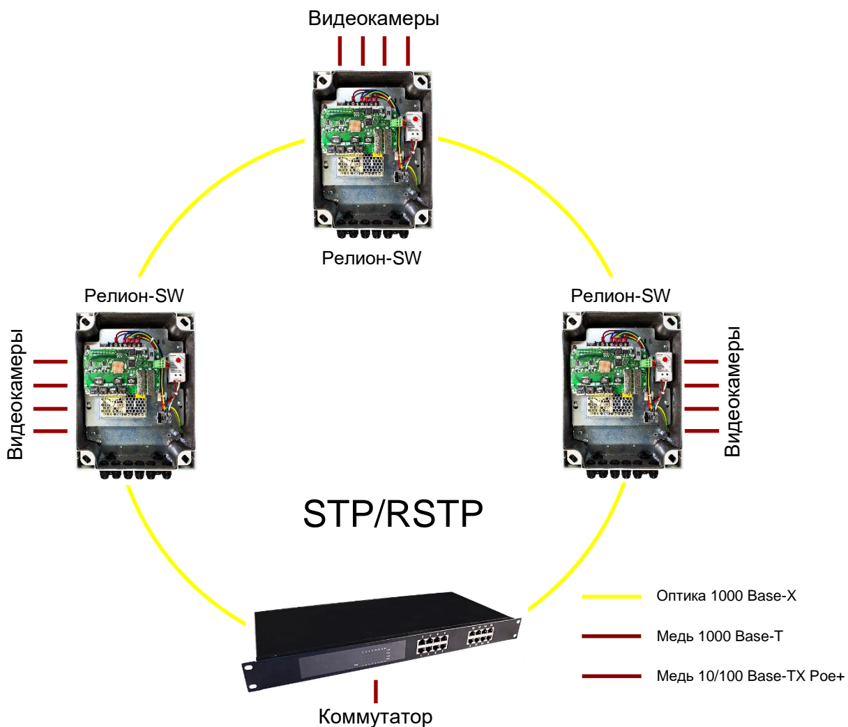
Рисунок 11. Подключение коммутаторов в топологию «линия»
