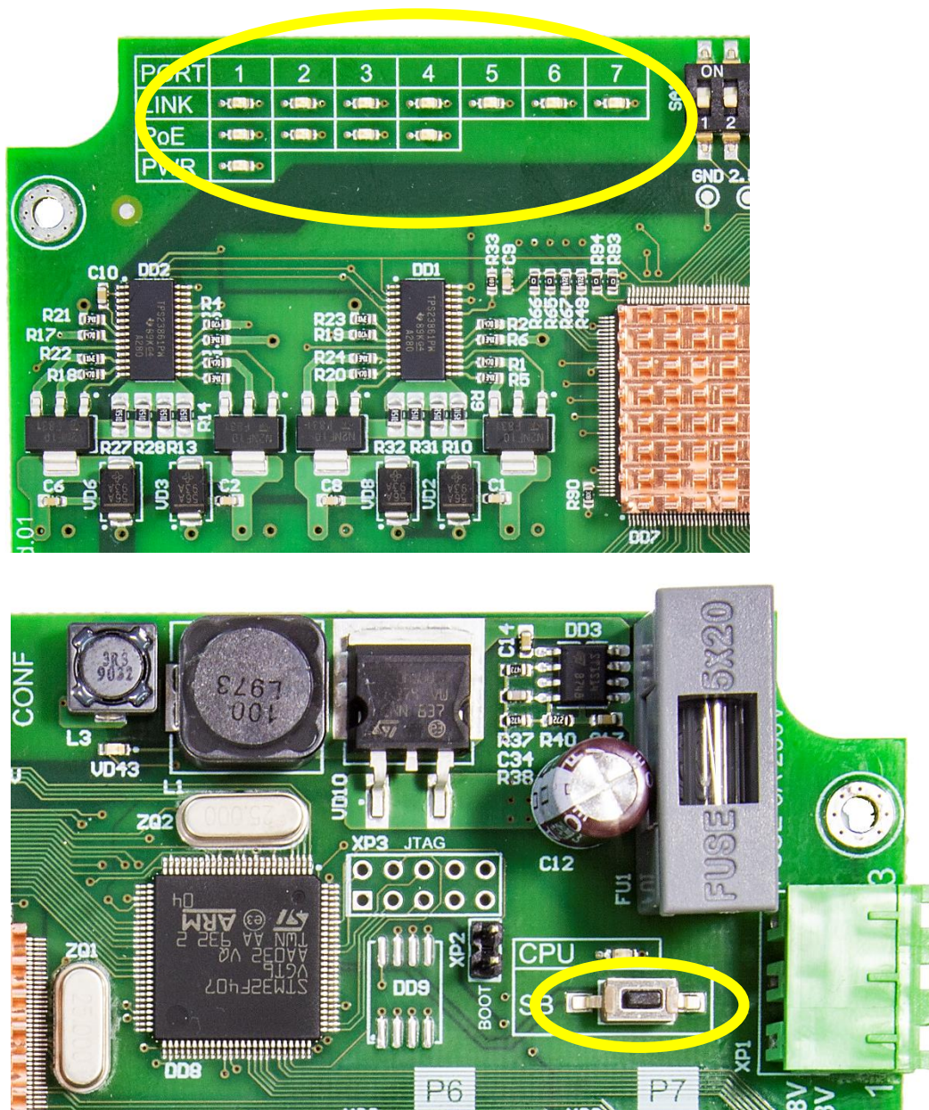
Рисунок 13. Расположение элементов индикации и настройки на плате коммутатора
