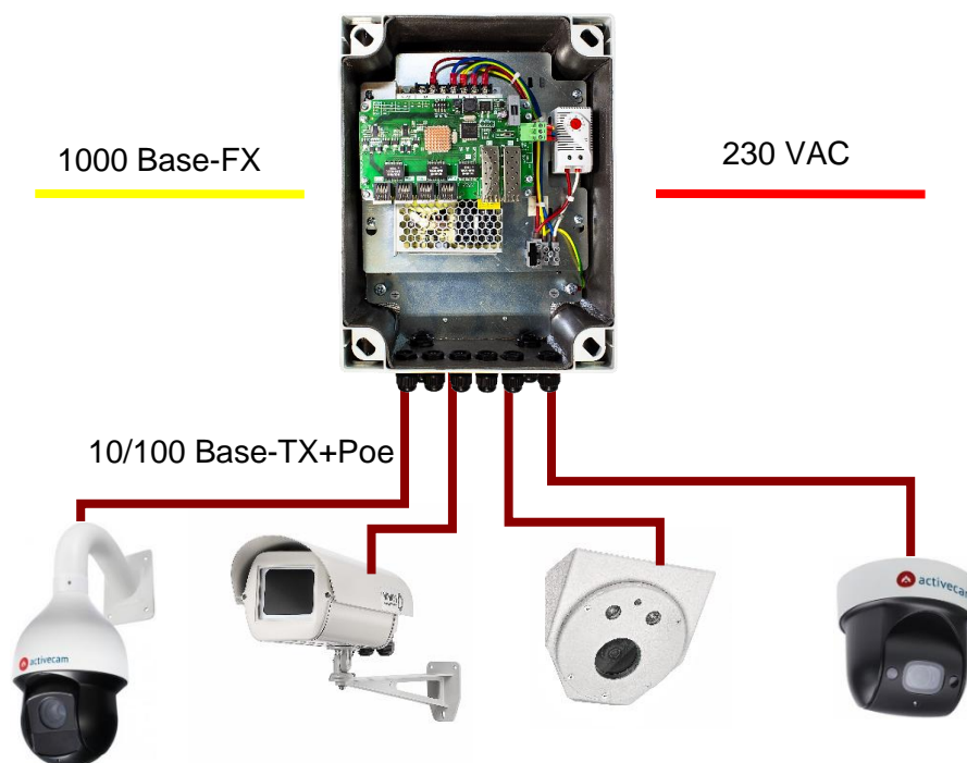
Рисунок 1. Типовая схема подключения коммутаторов по одному оптическому кабелю.
