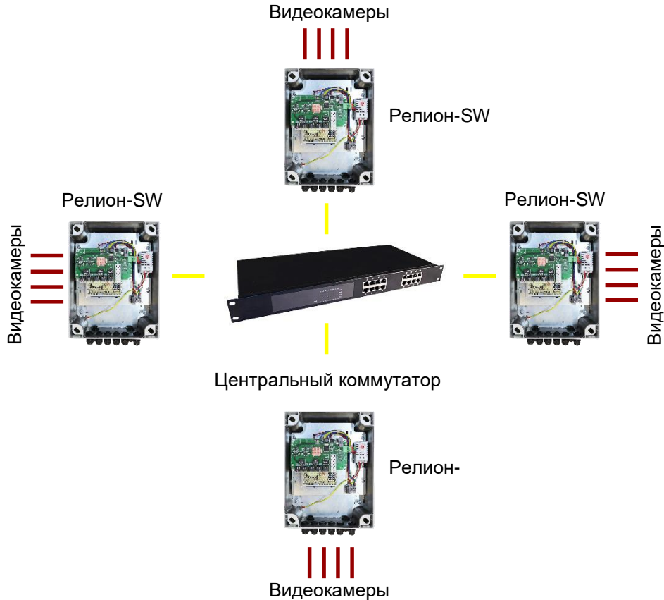
Рисунок 10. Подключение коммутаторов в топологию «звезда»
