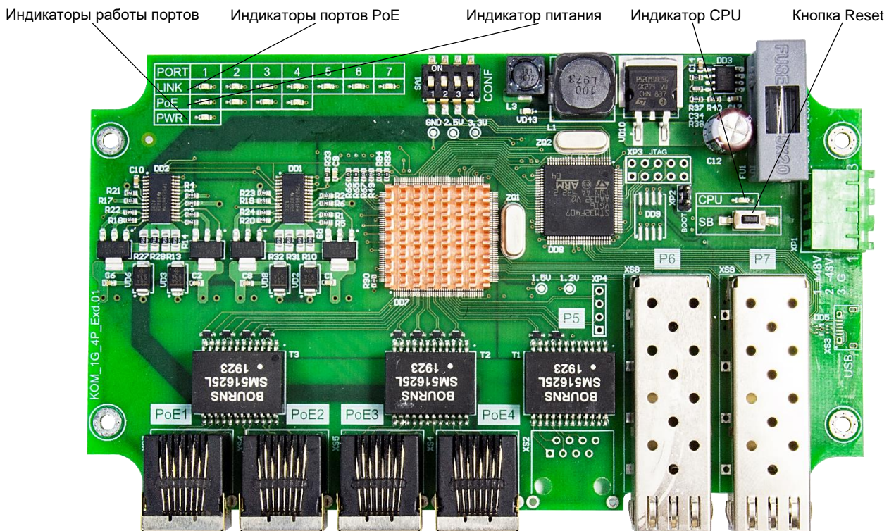
Рис. 8. Расположение элементов
