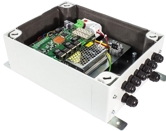
Рисунок 5. Вид изнутри
