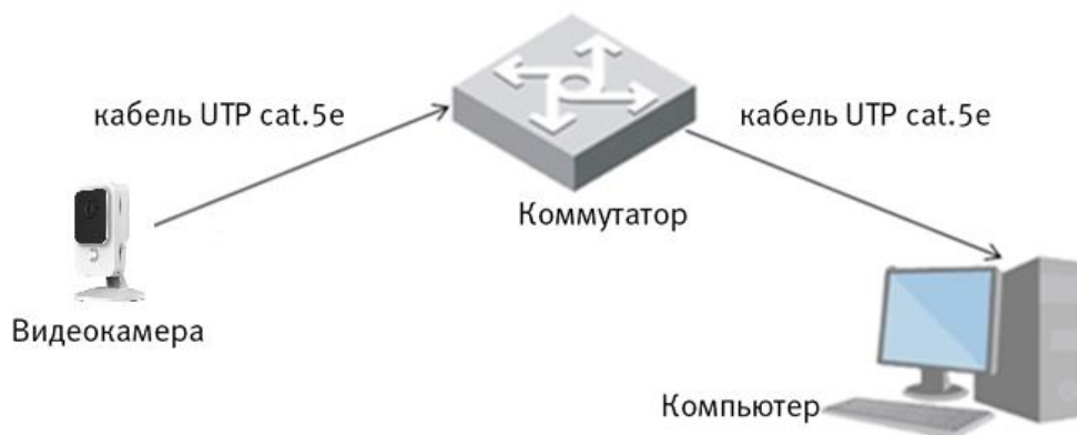
Рисунок 5.4 - Схема подключения видеокamеры к компьютеру через коммутатор
