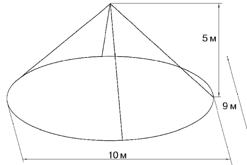
Рис.1 Вид зоны обнаружения ИК-канала
