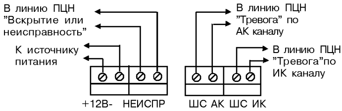
Рис. 4 Схема подключения извещателя
