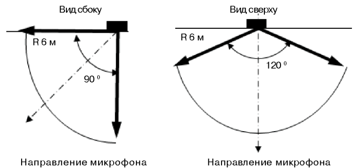
Рис. 2 Вид зоны обнаружения АК-канала
