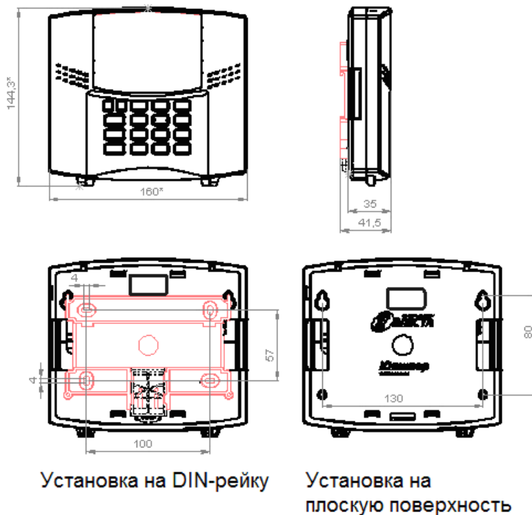
Рисунок 2. Габаритные и установочные размеры прибора
