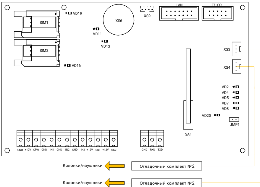
Рисунок 11. Схема подключения «Отладочного комплекта №2»
