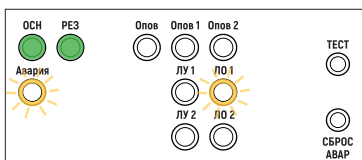
Рис. 81. Пример индикации на двухзональном БР после устранения неисправности в линии оповещения
