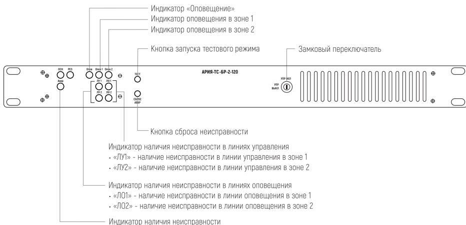
Рис. 7. Лицевая панель блока расширения АРЯ-ТС-EP-2-120.
