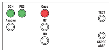
Рис. 48. Индикация на однозональном БР при трансляции сообщения с линейного входа
