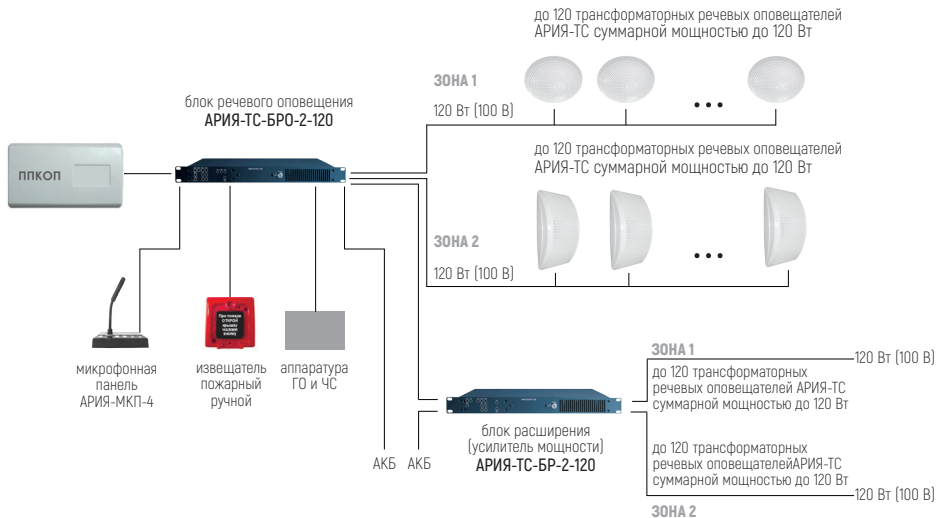
Рис. 1. Пример соединения оборудования в системе АРИА-ТС
