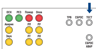
Рис. 31. Индикация режима «Тест» на однозональном БРО
