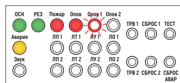
Рис. 83. Пример индикации при отсутствии в памяти двухзонального БРО сообщения для персонала или тревожного сообщения для зоны 1
