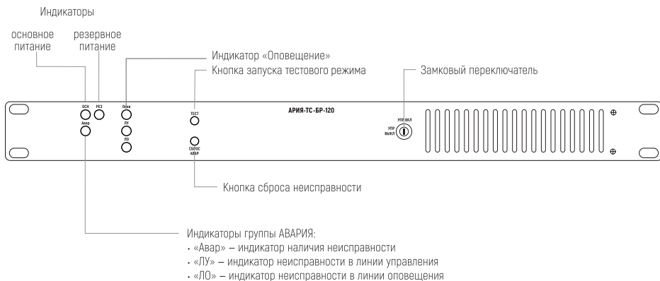
Рис.6. Лицевая панель блока расширения АРЯ-ТС-EP-120.
