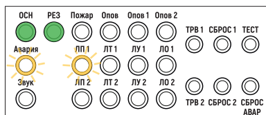
Рис. 61. Индикация после устранения неисправности в зоне 1 в двухзональном БРО
