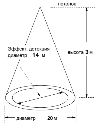
рис. 3 TLC-360 Диаграмма направленности детектора
