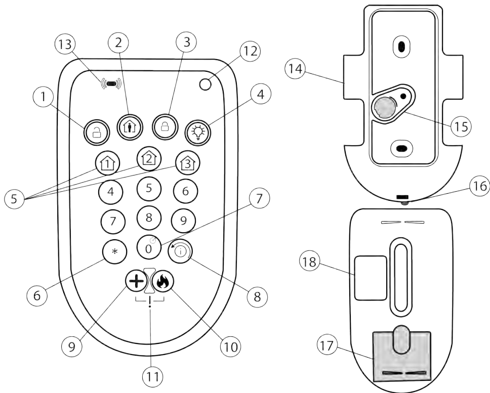
Рисунок 1: Компоненты клавиатуры
