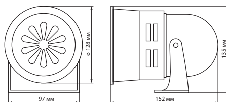
Рисунок 1. Габаритные и установочные размеры
