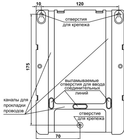
Рис.2 Присоединительные размеры
