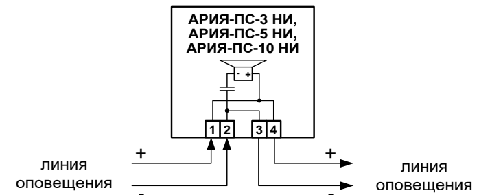
Рис.1. Схема подключения.
