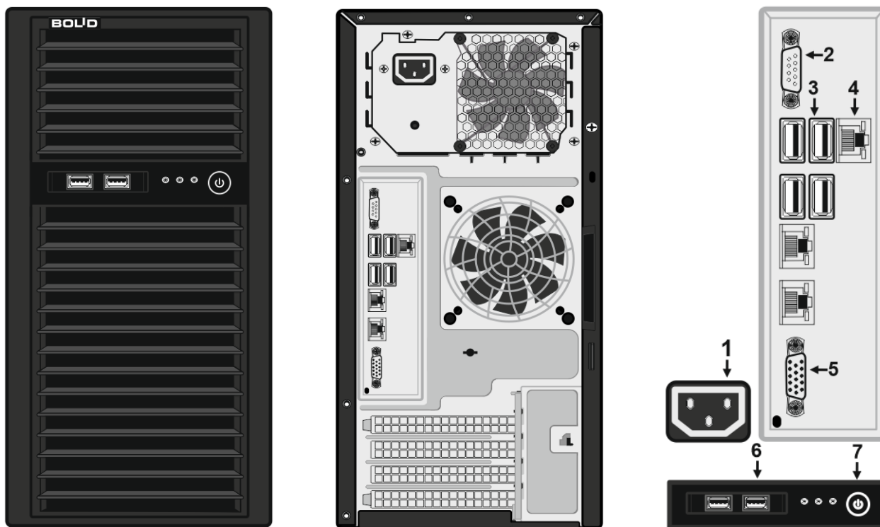
Рисунок 1. Конструкция системного блока.
