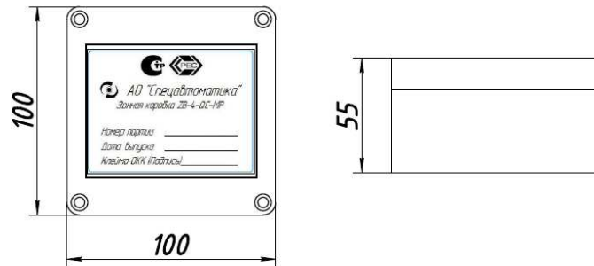
Рисунок 1. Общий вид зонной коробки ZB-4-QC-MP
