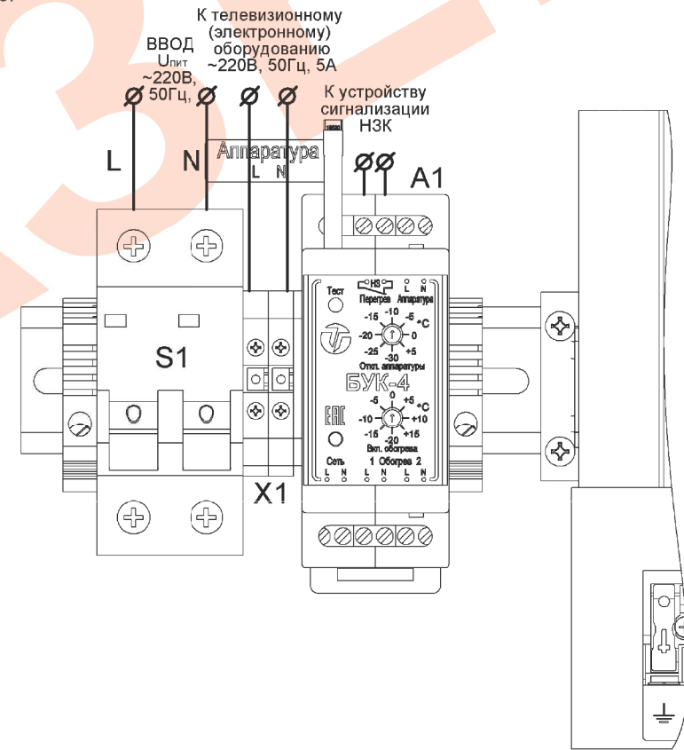
Рис.2. Подключение термощафа
